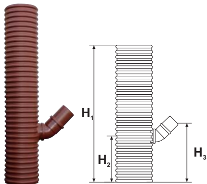
PP Rindestensbrønd med vandlås
